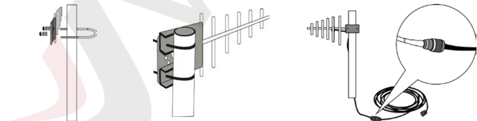
Пример установки всепогодной антенны типа «волновой канал» (антенна Яги)
